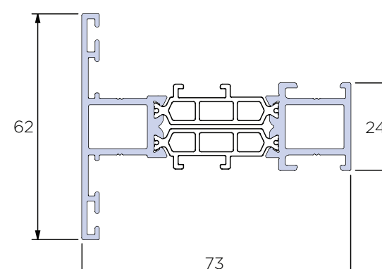
Slim Transom- Cleat Fix ACW81.444
