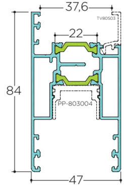
TV 80402 6,5m 845 gr/m Interlock Profile 25mm
