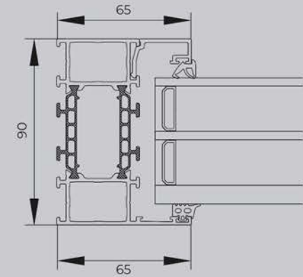
Sidelight
