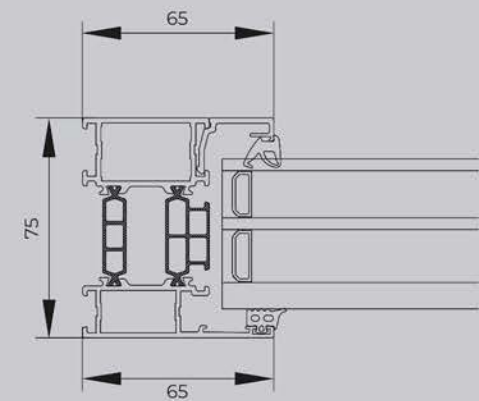
Sidelight
